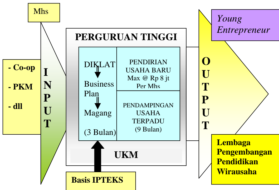
Gambar 1. Skema Program
